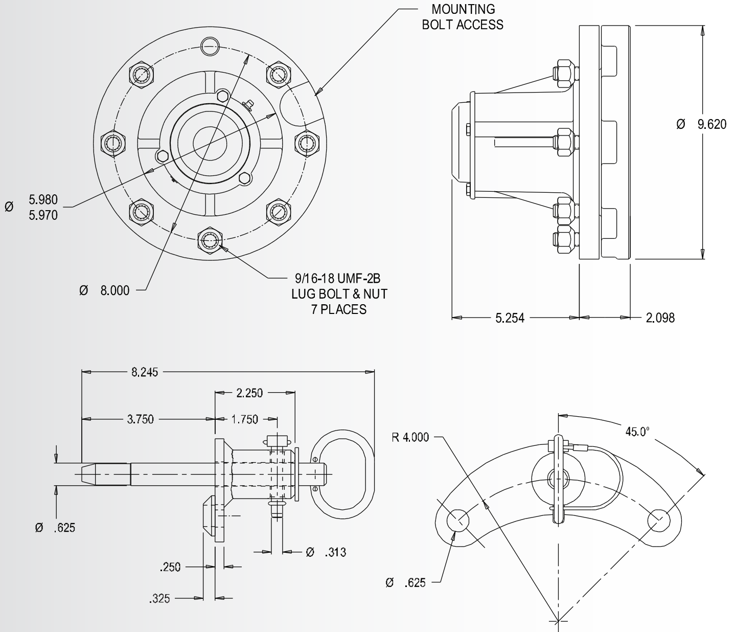
Moyeu Tractable BT4-B à boulonner et Assemblage et Goupille Charnière
